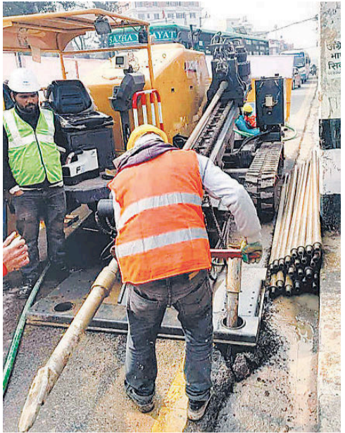
काठमाडौंमा होराइजेन्टल डाइरेक्सन ड्रिलिङ प्रविधिबाट तार फाइल तयार : कान्तिपुर
